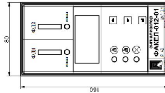
Габаритные размеры сигнализатора устройства контроля факела Факел-012-01
