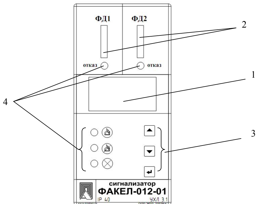
Рис.1. Лицевая панель сигнализатора Факел-012-01. 1 – ЖКИ; 2 – светодиодные линейки; 3 – кнопки; 4 – светодиоды.
