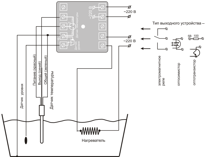
Схема электрическая подключения терморегулятора РАТАР-02.п/п – Ц3
