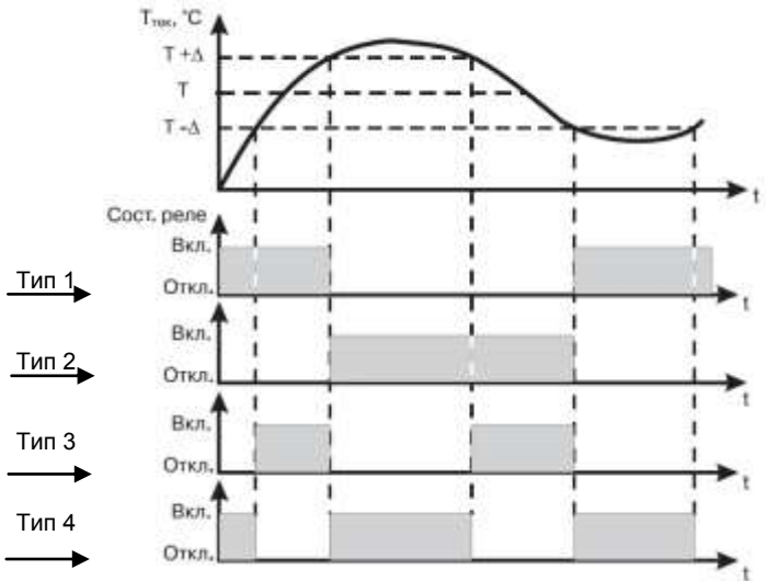
Рисунок 2 – Диаграммы работы выходного устройства терморегулятора РАТАР-02.п/п
