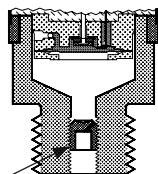
Демпфер пульсаций давления
